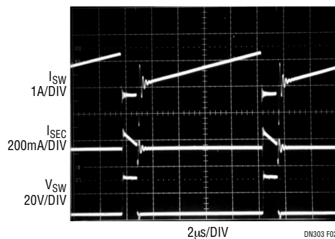
図2. V_{OUT}=300V 、 V_{CC}=V_{BAT}=3.3V でのスイッチング波形
