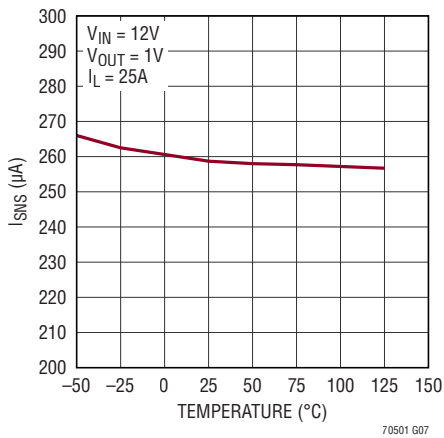
I_{SNS} と温度の関係
