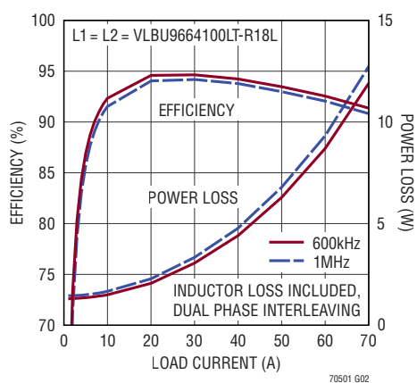
12V IN /1.8V OUT の効率
