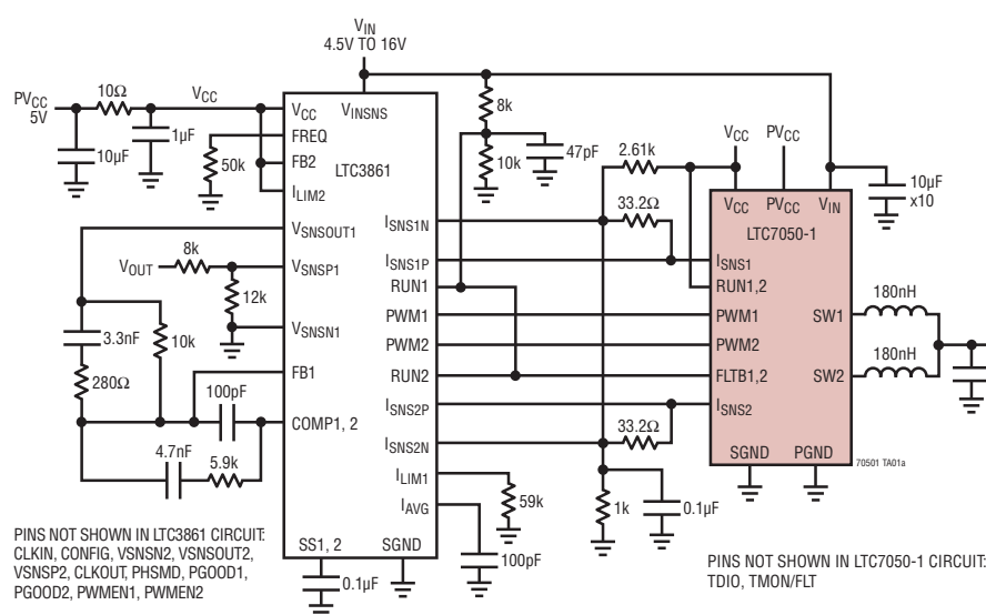
12VIN、1V/70A OUT 、1MHzのデュアルフェーズPOLコンバータ
