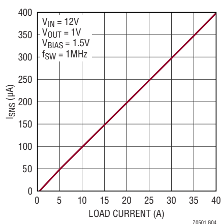
I SNS と負荷の関係
