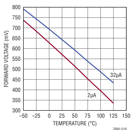
T_{\text{DIODE}} 順電圧と温度の関係
