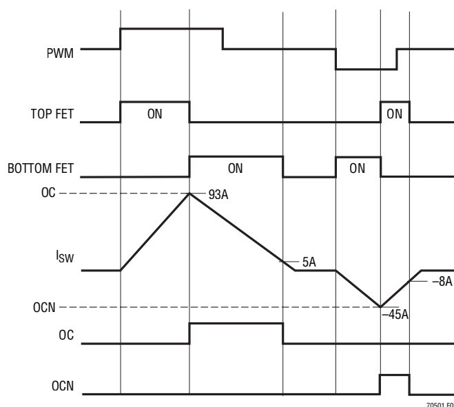
図3. 過電流状態
