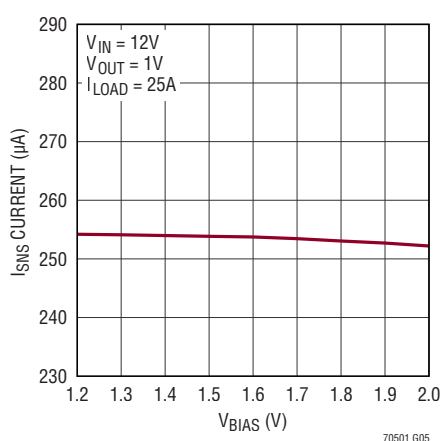
I SNS 電流とV BIAS の関係
