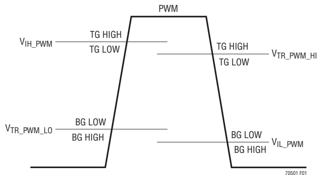
図1.3 ステート入力動作
