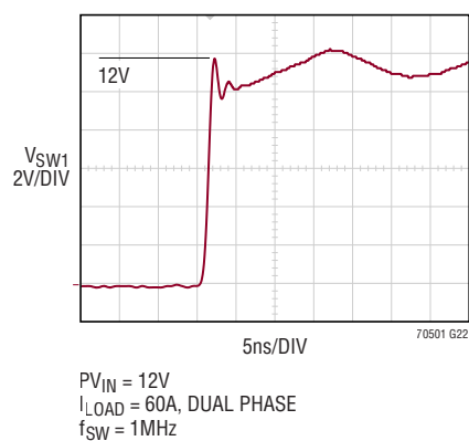
スイッチング時の立上がりエッジ
