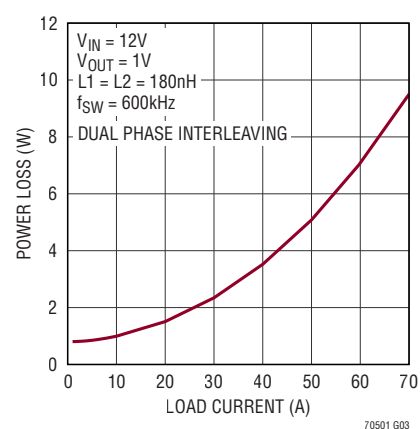
LTC7050-1 消費電力と負荷の関係
