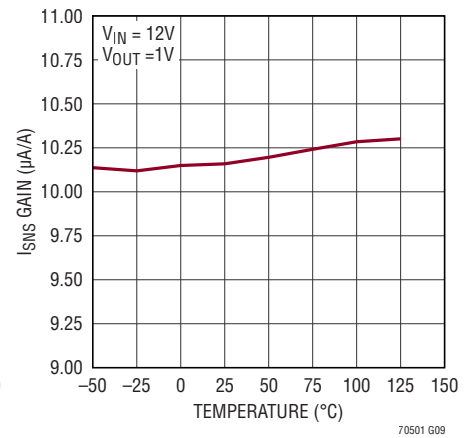
I_{SNS} ゲインと温度の関係
