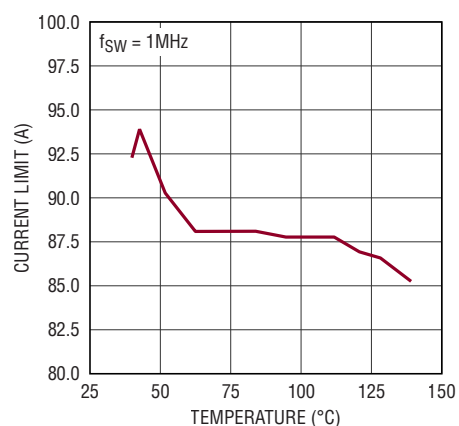
電流制限値と温度の関係
