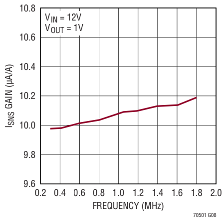
I_{SNS} ゲインと周波数の関係
