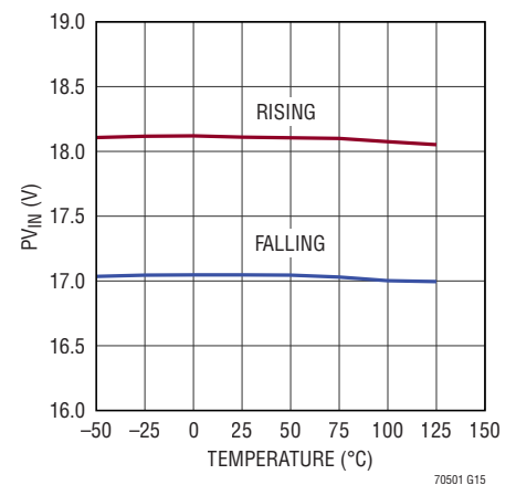
PV_{IN} OVLO と温度の関係
