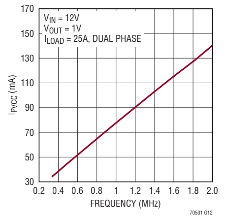
I_{PVCC} と周波数の関係
