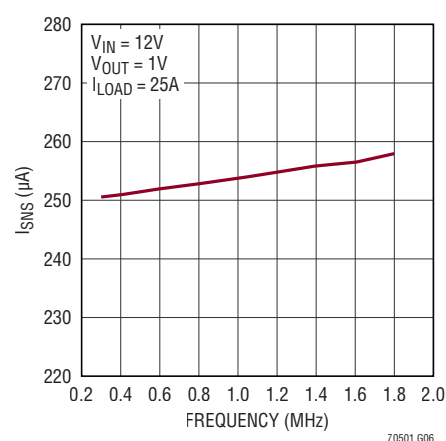
I SNS と周波数の関係
