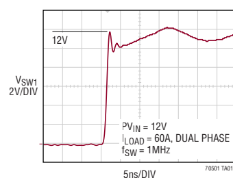
1MHz 時の V_{SW} 波形
