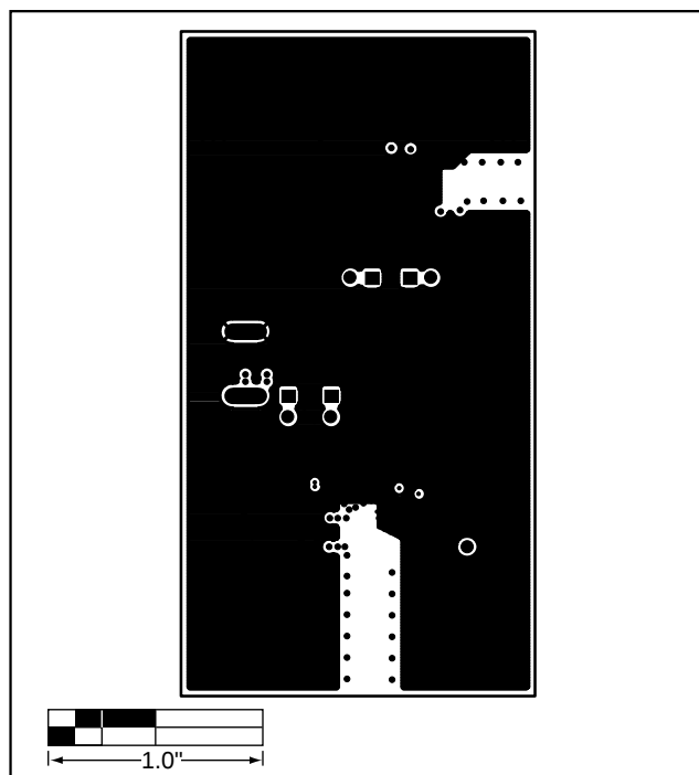
図4. MAX2251EVキットPC基板レイアウト (グランドプレーン)
