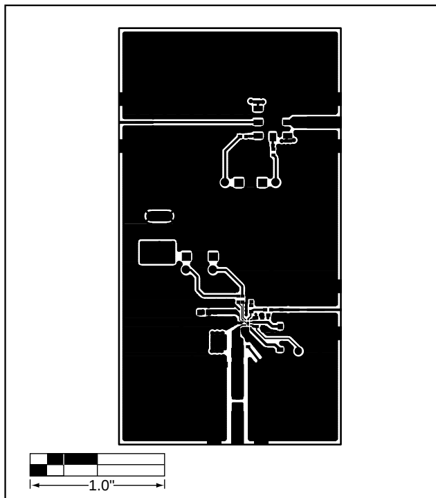
図3. MAX2251EVキットPC基板レイアウト(部品面側)
