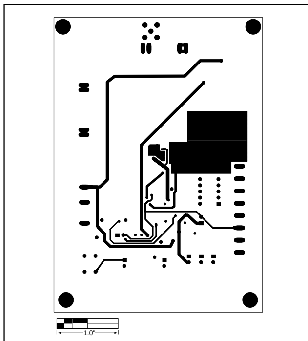
図7. MAX1711電圧ポジショニングEVキットのプリント基板レイアウト(ハンダ面側)
