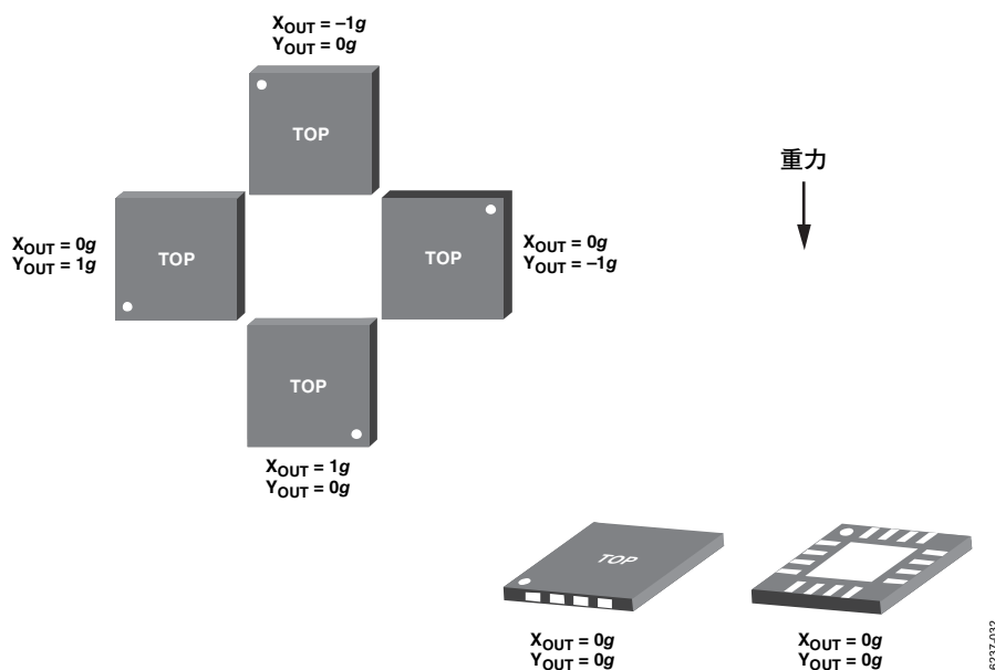
図32. 出力応答と重力方向の関係
