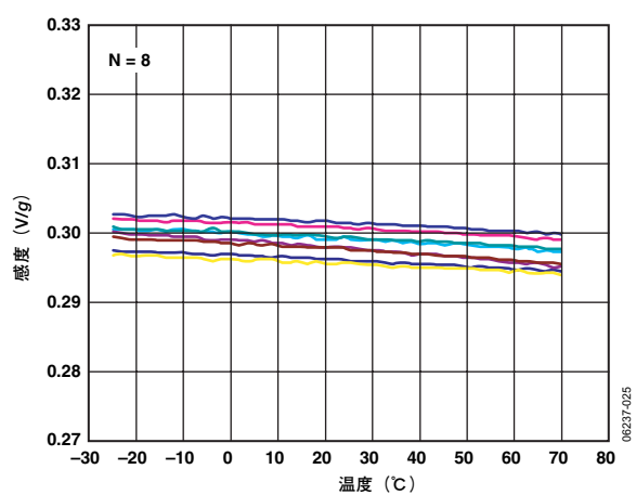
図25. X軸感度の温度特性 (8個のデバイスをPCボードにハンダ付け、 V_S=3V )
