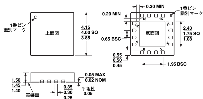
図33. 16ピン・リード・フレーム・チップ・スケール・パッケージ [LFCSP_LQ] 4mm×4mmボディ、クワッド (CP-16-5) 寸法単位：mm
