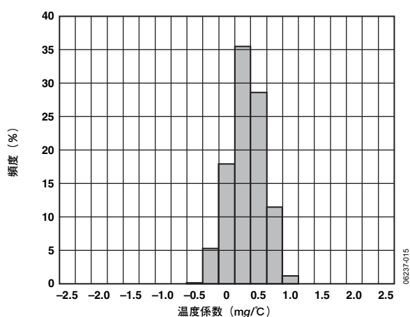
図15. Y軸のゼロgバイアス温度係数 ( V_S=5V )
