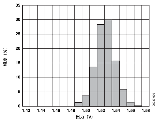
図9. Y軸のゼロgバイアス (25°C、 V_S=3V )
