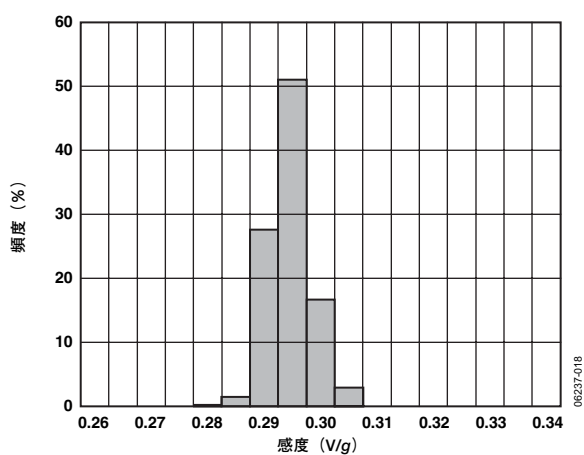
図18. X軸の感度 (25°C、 V_S=3V )
