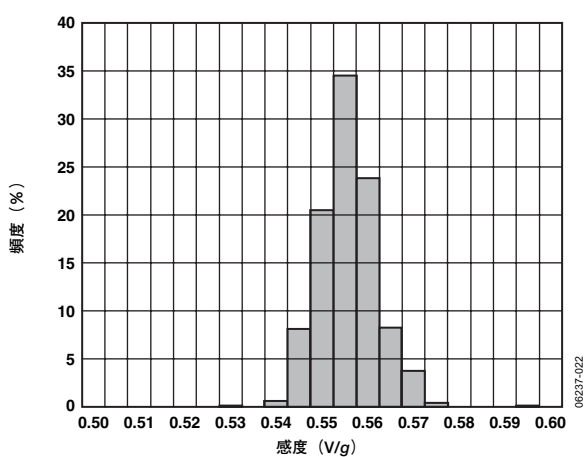
図22. Y軸の感度 (25°C、 V_S=5V )
