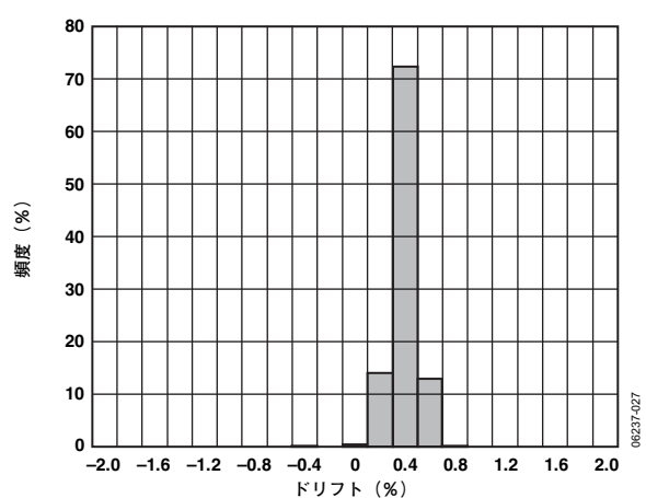
図27. Y軸感度の温度特性ドリフト ( V_S=5V )
