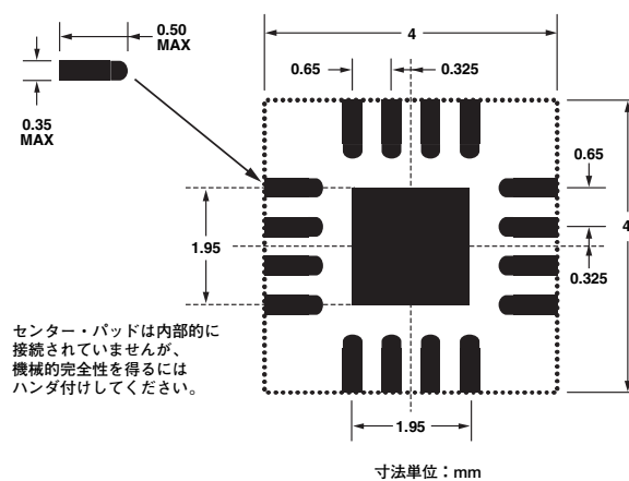
図4. 推奨するPCボードのレイアウト
