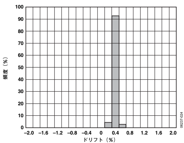
図24. X軸感度の温度ドリフト ( V_S=5V )
