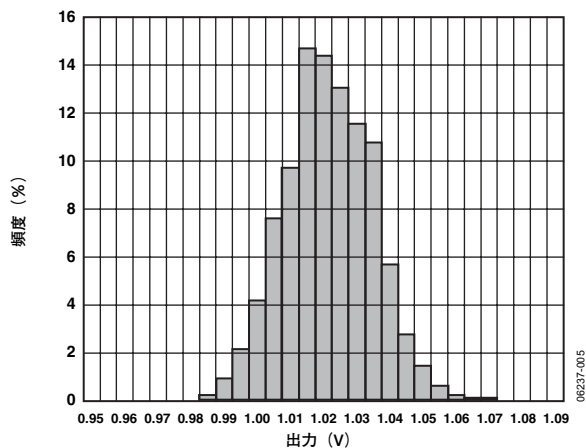
図5. X軸のゼロgバイアス (25°C、 V_S=2V )
