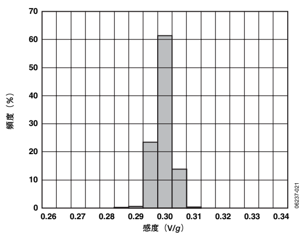
図21. Y軸の感度 (25°C、 V_S=3V )
