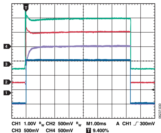
図30. 代表的なターンオン時間 ( C_X 、 C_Y=0.0047\mu\text{F} 、 V_S=3\text{V} )
