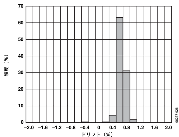
図26. Y軸感度の温度ドリフト ( V_S=3V )
