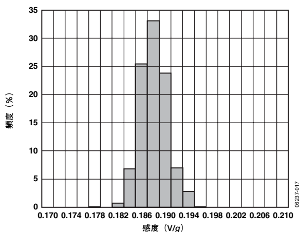
図17. X軸の感度 (25°C、 V_S=2V )
