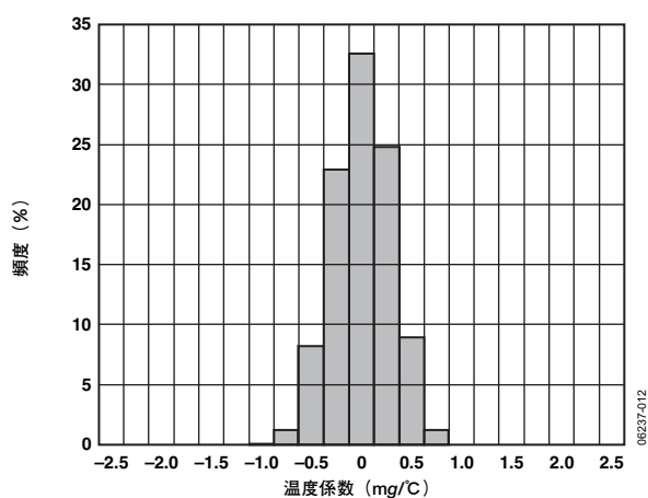
図12. X軸のゼロgバイアス温度係数 ( V_S=5V )
