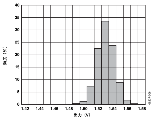
図6. X軸のゼロgバイアス (25°C、 V_S=3V )
