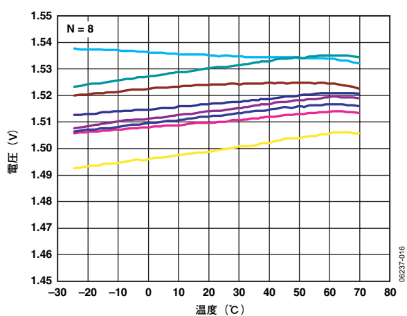
図16. Y軸のゼロgバイアスの温度特性 (8個のデバイスをPCボードにハンダ付け、 V_S=3V )
