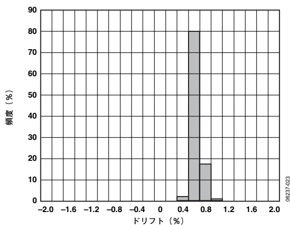
図23. X軸感度の温度ドリフト ( V_S=3V )
