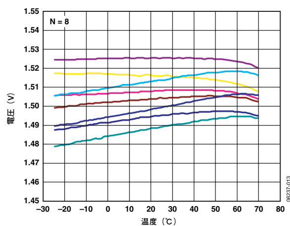
図13. X軸のゼロgバイアスの温度特性 (8個のデバイスをPCボードにハンダ付け、 V_S=3V )
