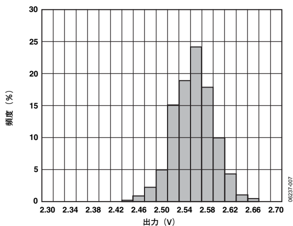
図7. X軸のゼロgバイアス (25°C、 V_S=5V )
