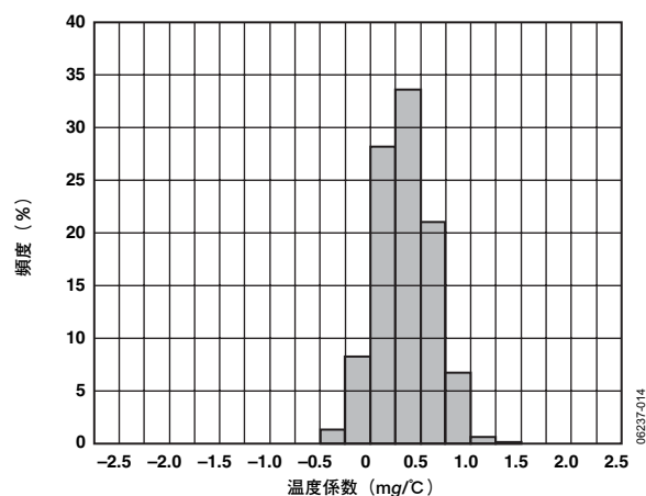
図14. Y軸のゼロgバイアス温度係数 ( V_S=3V )
