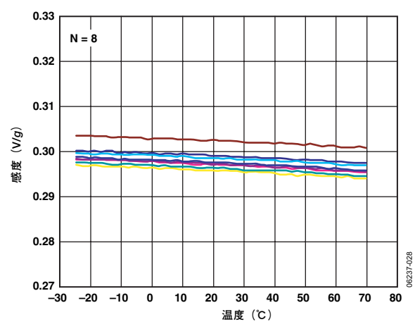
図28. Y軸感度の温度特性 (8個のデバイスをPCボードにハンダ付け、 V_S=3V )
