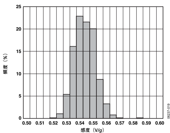
図19. X軸の感度 (25°C、 V_S=5V )
