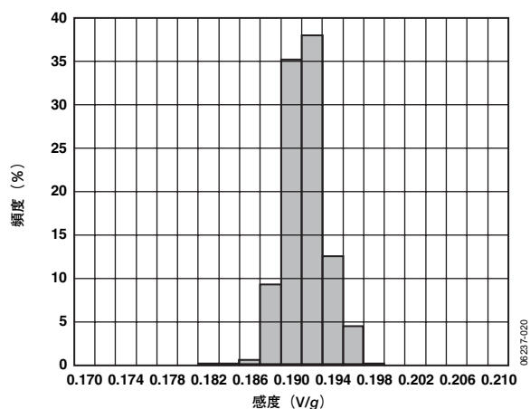
図20. Y軸の感度 (25°C、 V_S=2V )
