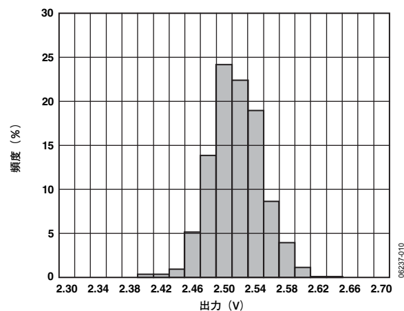
図10. Y軸のゼロgバイアス (25°C、 V_S=5V )
