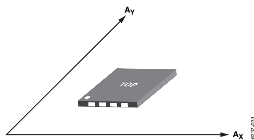
図31. 加速度検出軸方向 (検出軸に沿って加速されると、対応する出力電圧が増加)
