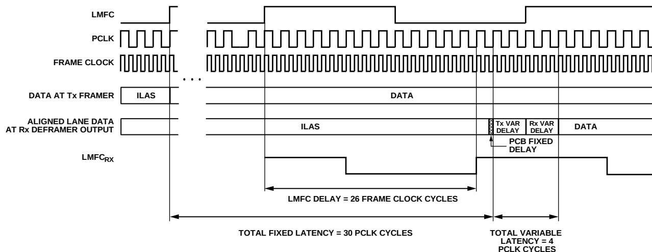
図 40. LMFC 遅延計算例
