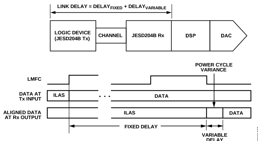
図 37. JESD204B のリンク遅延 = 固定遅延 + 可変遅延
