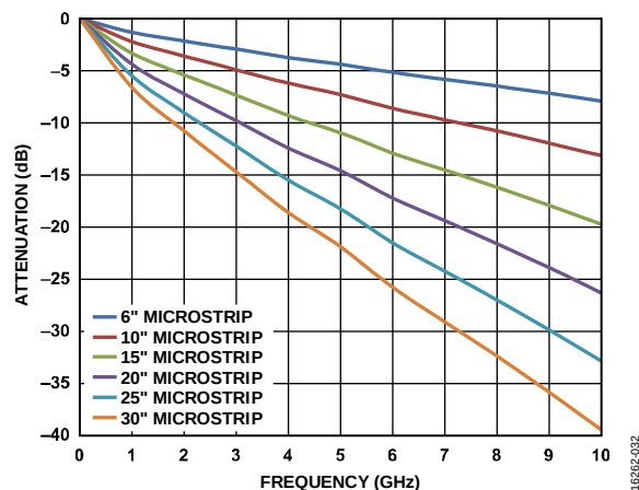
図 32. FR4 の 50 Ω マイクロストリップの挿入損失
