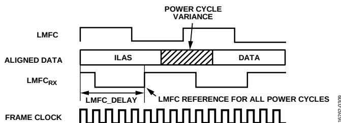
図 39. LMFC 周期より大きいリンク遅延を補償する LMFC_DELAY_x
