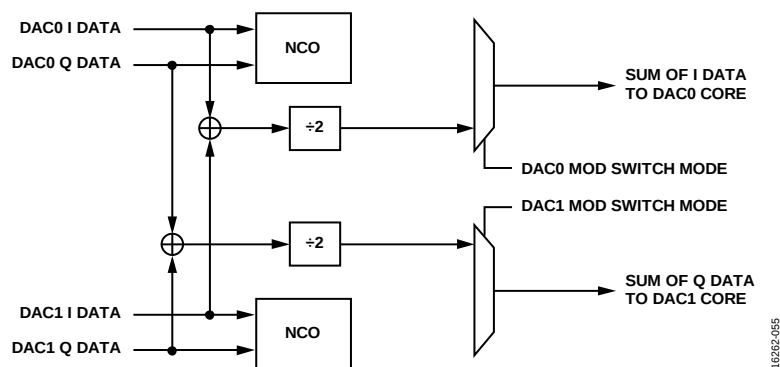
図 55. モード 1 —DAC0 = I0 + I1、DAC1 = Q0 + Q1
