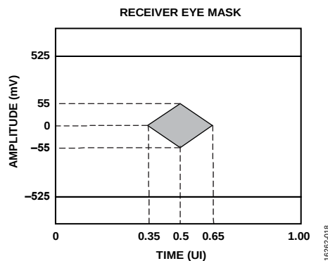
図 28. レシーバー・アイ・マスク
