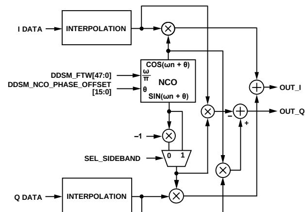
図 53. NCO 変調器のブロック図
