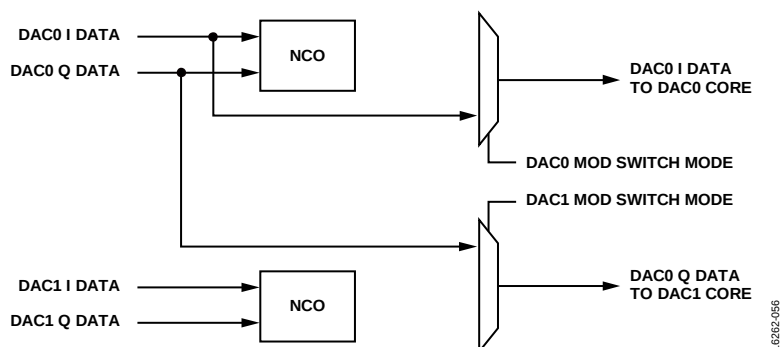
図 56. モード 2 —DAC0 = I0、DAC1 = Q0
