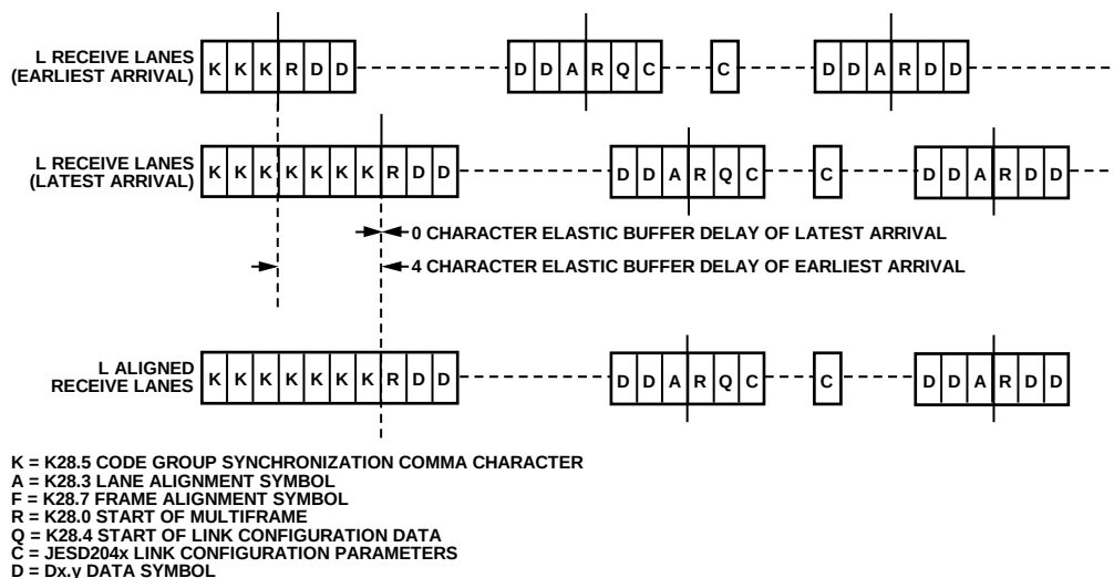
図 34. ILAS でのレーン・アライメント
