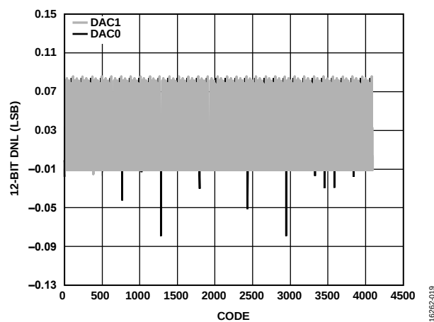
図 19. DNL - I_{OUTFS} = 20 \text{ mA} 、12 ビット分解能
