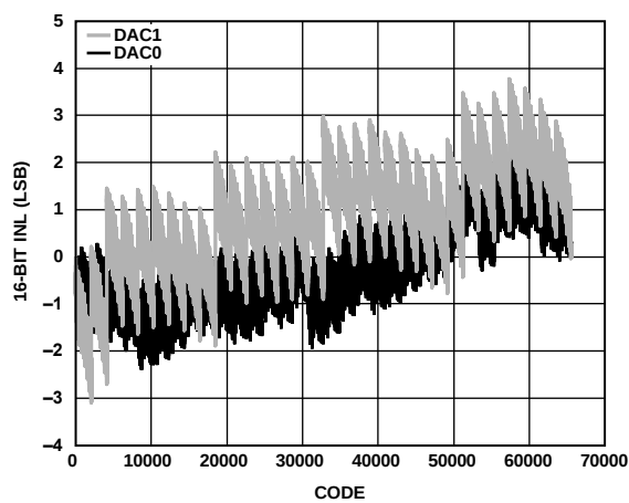
図 16. INL - I_{OUTFS} = 20 \text{ mA} 、16 ビット分解能
