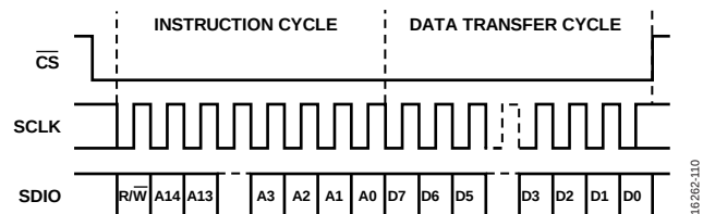
図 22. シリアル・レジスタ・インターフェースのタイミング - MSB ファースト、レジスタ 0x000、ビット 6 およびビット 1 = 0
