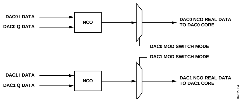
図 54. モード 0 —DAC0 = I0、DAC1 = I1
