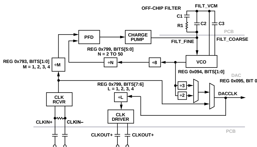
図 65. DAC PLL とクロック・パスのブロック図
