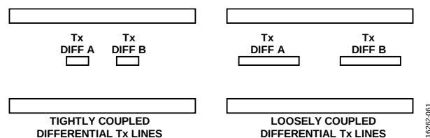
図 61. 狭い間隔で配置した差動パターンと 広い間隔で配置した差動パターン
