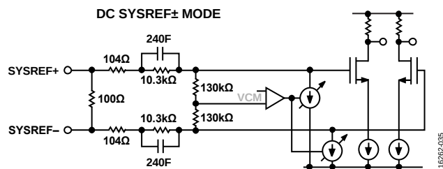
図 35. DC カップリングした SYSREF± レシーバー回路
