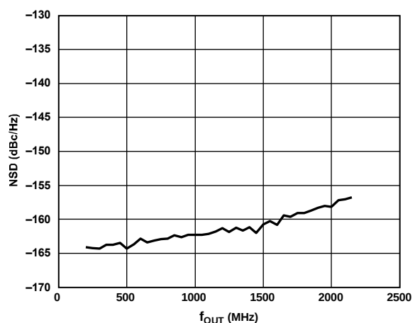
図 10. 70 MHz で測定したシングル・トーン NSD と f_{OUT} の関係: f_{DAC} = 5.89824 GHz、12 ビット分解能、シャッフル・オン
