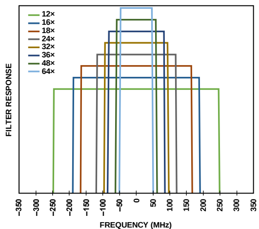
図 44. 合計インターポレーション・レートの帯域応答 - 6 GHz DAC レート、16 ビット分解能で 8×、12×、16×、18×、24×、32×、36×、48×、64×
