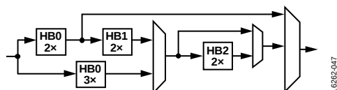
図 47. チャンネル・インターポレーション・ハーフバンド・フィルタのブロック図
