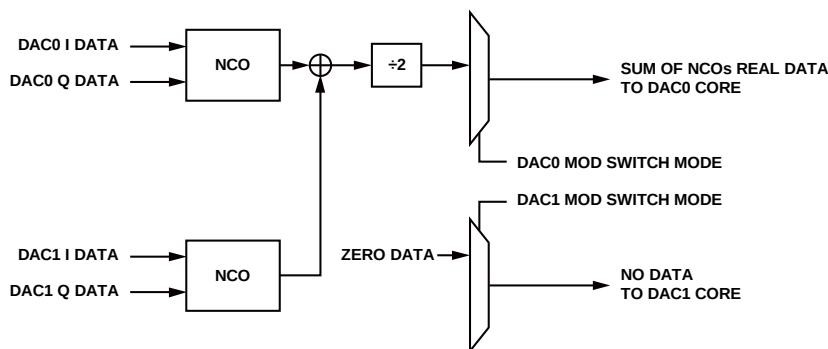
図 57. モード 3 —DAC0 = I0 + I1、DAC1 = 0
