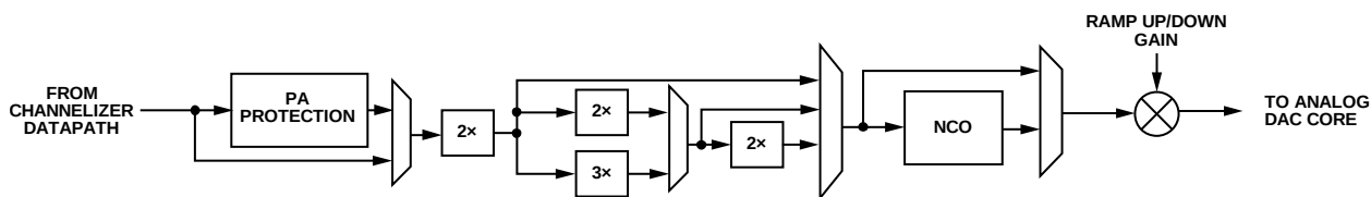
図 49. メイン DAC 出力ごとのメイン・デジタル・データパスのブロック図
