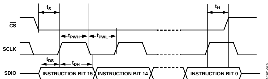
図 25. シリアル・ポート・レジスタの書込みタイミング図
