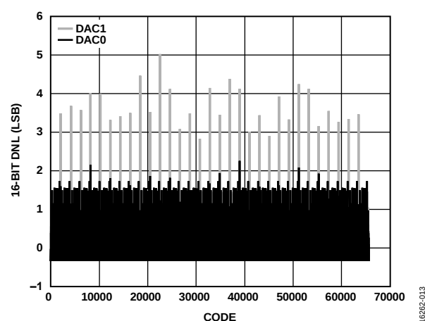
図 13. DNL - I_{OUTFS} = 26 mA、16 ビット分解能
