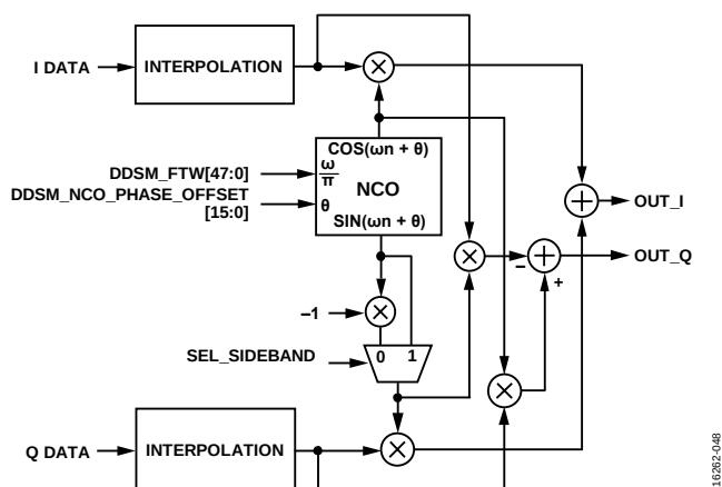
図 48. NCO 変調器のブロック図
