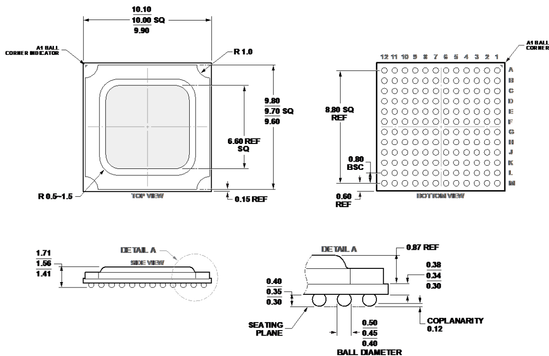
図 67. 熱強化型 144 ボール BGA [BGA_ED] (BP-144-1) 寸法: mm
