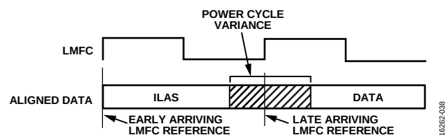
図 38. リンク遅延が LMFC 周期より大きい例
