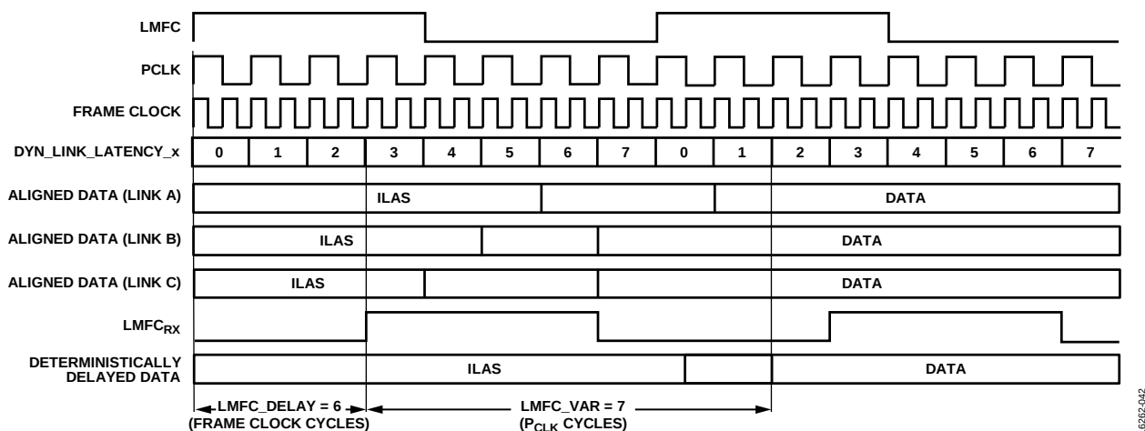
図 42. マルチリンク同期設定、導出方法の例
