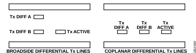
図 60. ブロードサイド法とコプラナー法による 差動ストリップライン配線
