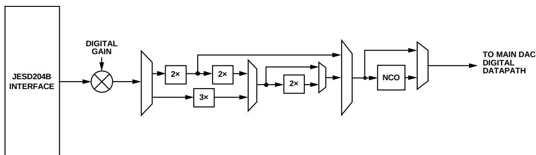
図 46. メイン DAC 出力ごとのチャンネル・デジタル・データパスのブロック図
