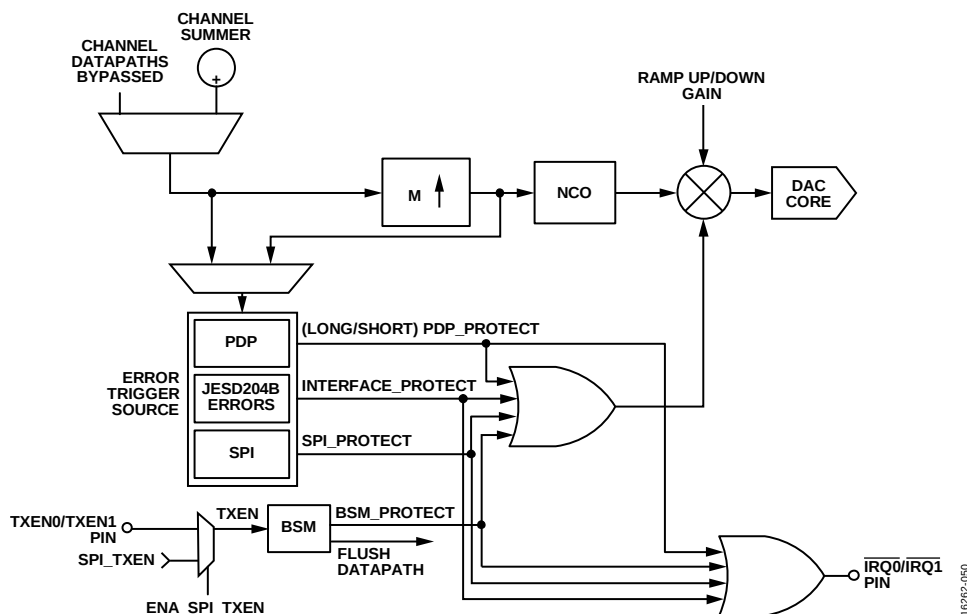
図 50. ダウンストリーム保護トリガのブロック図
