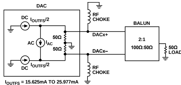
図 66. 等価 DAC 出力回路と推奨 DAC 出力回路
