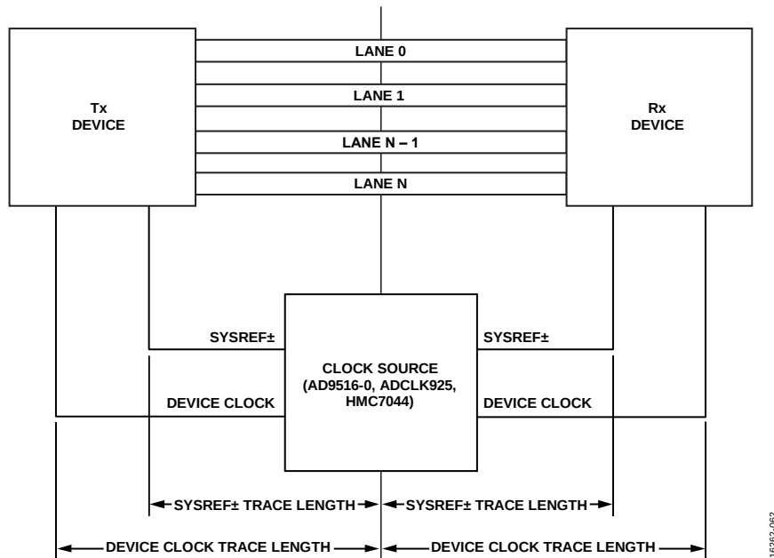
図 62. SYSREF ± 信号とデバイス・クロックのパターン長
