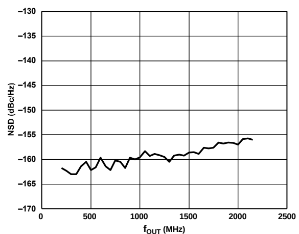
図 11. f_{OUT} から 10 % のオフセットで測定したシングル・トーン NSD と f_{OUT} の関係: f_{DAC} = 5.89824 GHz、12 ビット分解能、シャッフル・オン
