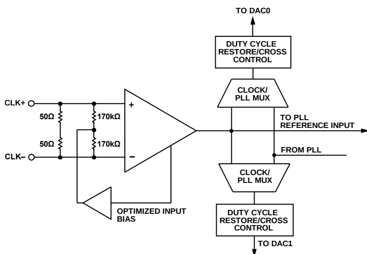
図 63. クロック・レシーバー入力の簡略等価回路
