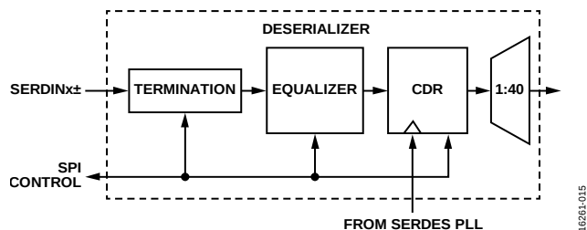
図 27. デシリアライザのブロック図
