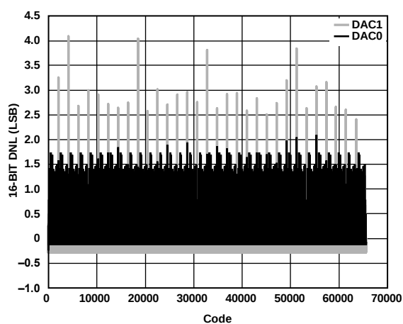
図 15. DNL - I_{OUTFS} = 20 \text{ mA} 、16 ビット分解能
