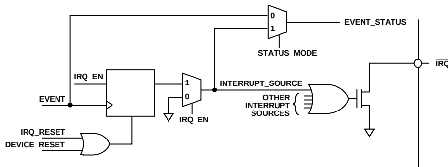
図 58. \overline{\text{IRQx}} 回路の簡略図
