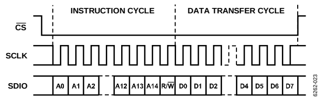
図 23. シリアル・レジスタ・インターフェースのタイミング - LSB ファースト、レジスタ 0x000、ビット 6 およびビット 1 = 1
