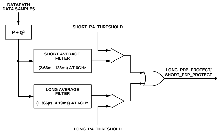
図 51. PDP のブロック図
