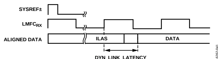
図 41. DYN_LINK_LATENCY_x の図
