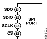
図 21. シリアル・ポート・インターフェース・ピン (144 ボール BGA_ED)
