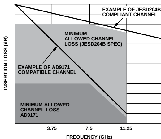
図 30. 許容挿入損失
