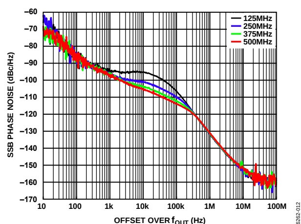
図 12. 単側波帯 (SSB) 位相ノイズと f_{OUT} オフセット - 異なる PFD 周波数での関係: f_{DAC} = 6 GHz、 f_{OUT} = 1.8 GHz、PLL オン、PLL リファレンス・クロック = PFD 周波数
