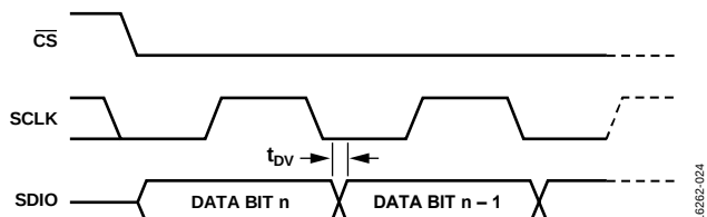
図 24. シリアル・ポート・レジスタの読出しタイミング図
