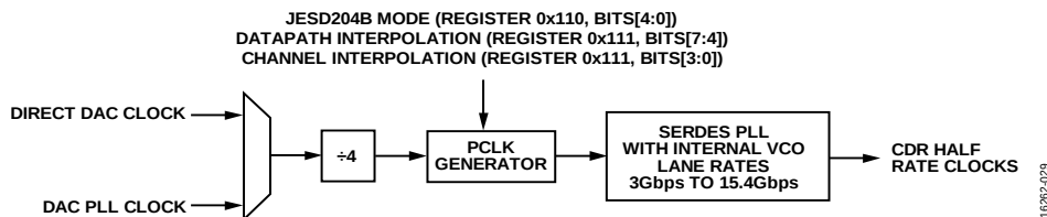
図 29. VCO 分周器ブロックを含む SERDES PLL シンセサイザのブロック図
