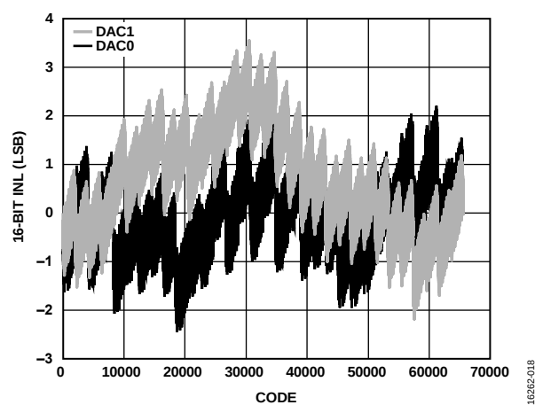
図 18. INL - I_{OUTFS} = 15.6 \text{ mA} 、16 ビット分解能
