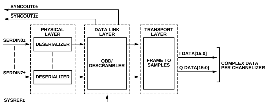
図 26. シリアル・リンク・レシーバーの機能ブロック図
