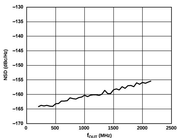
図 9. f_{OUT} から 10 % のオフセットで測定したシングル・トーン NSD と f_{OUT} の関係: f_{DAC} = 5.89824 GHz、16 ビット分解能、シャッフル・オン
