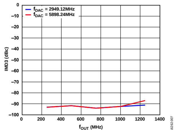
図 7. IMD3 と f_{OUT} - 異なる f_{DAC} (モード 0) での関係: チャンネル・インターポレーション 2 \times 、メイン・インターポレーション 8 \times 、1 MHz トーン間隔
