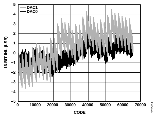
図 14. INL - I_{OUTFS} = 26 mA、16 ビット分解能
