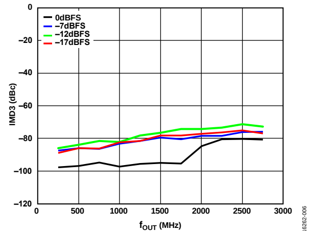
図 6. IMD3 と f_{OUT} - 異なるデジタル・スケール (モード 0) での関係: 6 GHz DAC サンプル・レート、チャンネル・インターポレーション 2 \times 、メイン・インターポレーション 8 \times 、1 MHz トーン間隔
