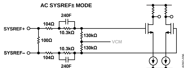
図 36. AC カップリングした SYSREF± レシーバー回路
