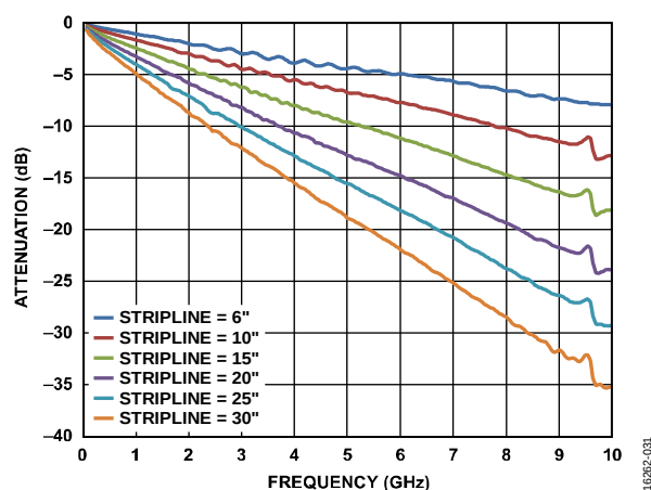
図 31. FR4 の 50 Ω ストリップラインの挿入損失
