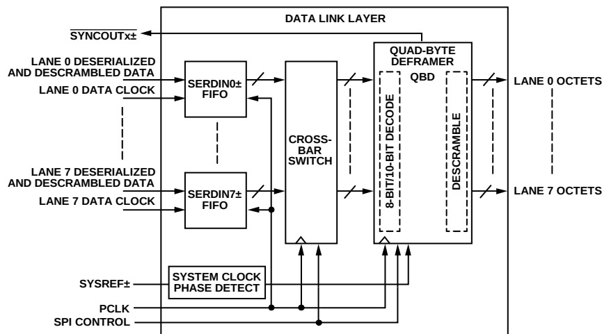
図 33. データ・リンク層のブロック図
