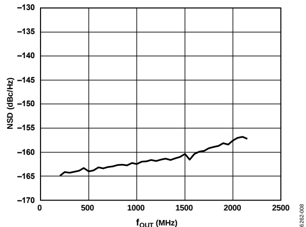
図 8. 70 MHz で測定したシングル・トーン NSD と f_{OUT} の関係: f_{DAC} = 5.89824 GHz、16 ビット分解能、シャッフル・オン
