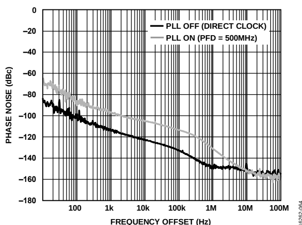
図 64. 位相ノイズと周波数オフセット - 直接クロックと PLL の位相ノイズ、6 GHz DAC サンプル・レート、1.8 GHz 出力周波数
