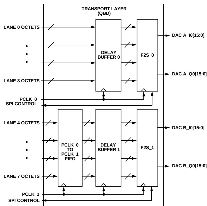
図 43. トランスポート層のブロック図
