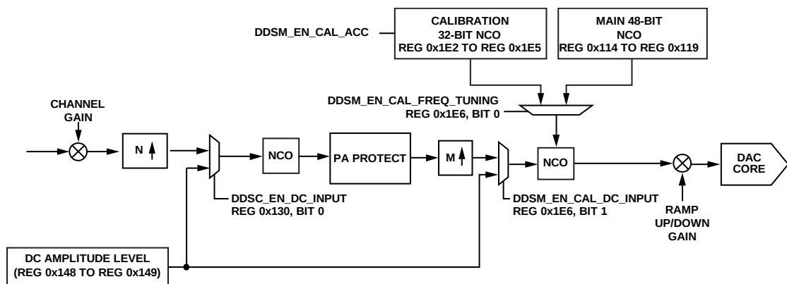
図 45. NCO オンリー・モードにおける DC 振幅注入のブロック図
