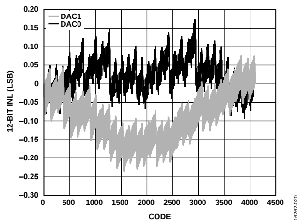
図 20. INL - I_{OUTFS} = 20 \text{ mA} 、12 ビット分解能
