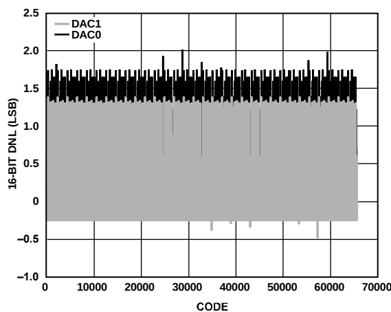
図 17. DNL - I_{OUTFS} = 15.6 \text{ mA} 、16 ビット分解能
