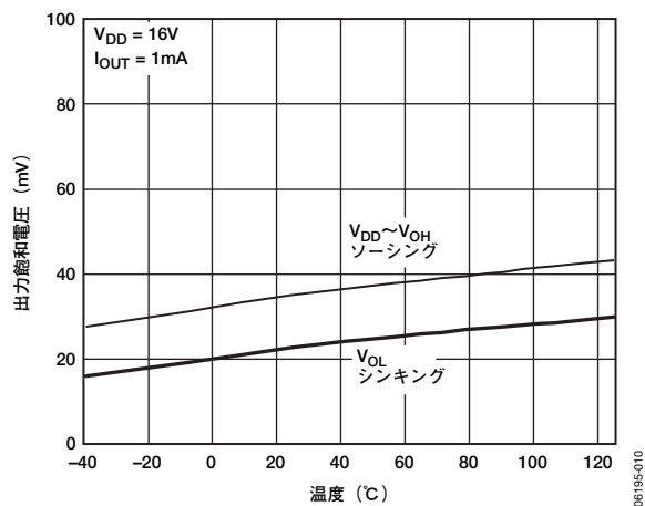
図12. 出力飽和電圧の温度特性
