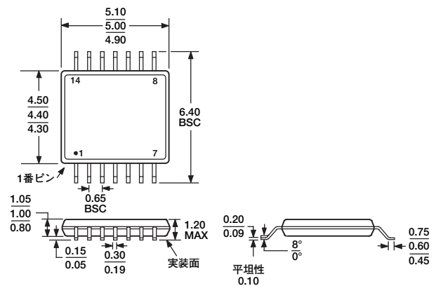
図43. 14ピン薄型シュリンク・スモール・アウトライン・ パッケージ [TSSOP] (RU-14) 寸法単位: mm
