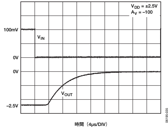
図37. 負の過負荷復帰時間
