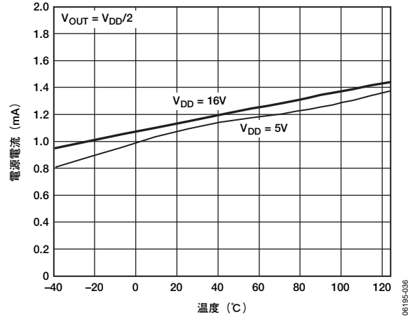
図38. 電源電流の温度特性
