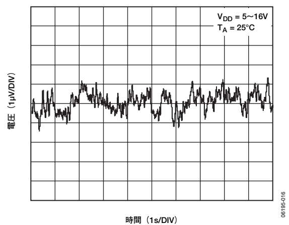
図18. 0.1～10Hzの電圧ノイズ
