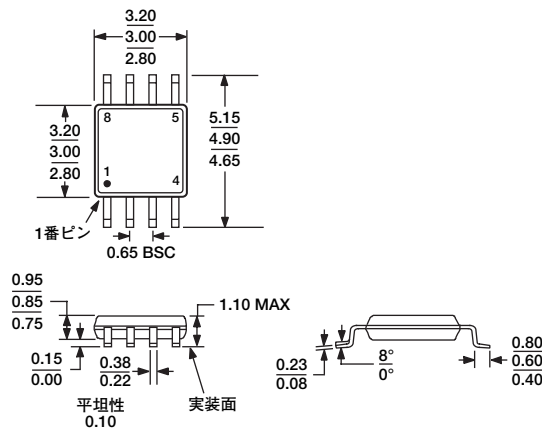
図42. 8ピン・ミニ・スモール・アウトライン・パッケージ [MSOP] (RM-8) 寸法単位: mm
