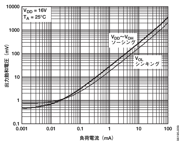
図11. 負荷電流 対 出力飽和電圧
