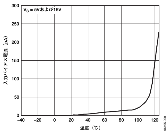
図10. 入力バイアス電流の温度特性
