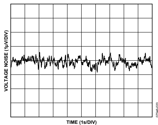
図 22. 0.1 Hz～10 Hz の電圧ノイズ、出力換算
