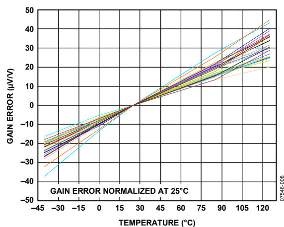
図 9. ゲイン誤差の温度特性、 25^\circ\text{C} で正規化
