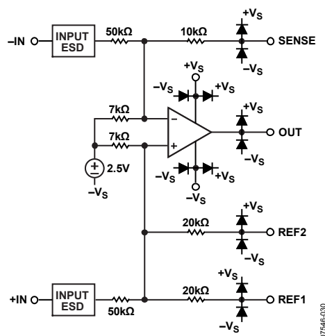
図 31. AD8275 の簡略化した回路図
