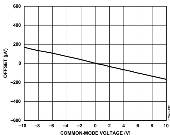
図 32. レール to レール入力の一般的なアンプにあるクロスオーバー歪みは AD8275 にはありません
