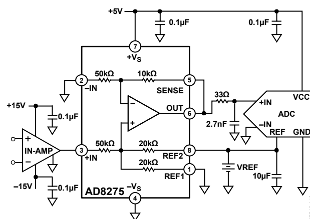
図 43. データ・アキュイジション・システムでのレベル変換
