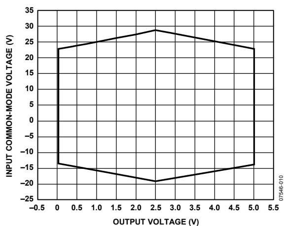
図 11.入力コモン・モード電圧対出力電圧、無負荷
