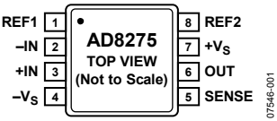
図 4. ピン配置
