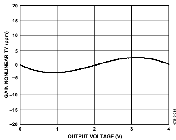
図 16.ゲイン非直線性、 R_L = 600\ \Omega 、 2\ \text{k}\Omega 、 10\ \text{k}\Omega
