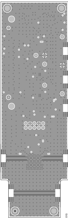
Figure 15. ADMV8502-EVALZ Layer 2
