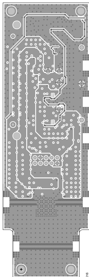
Figure 16. ADMV8502-EVALZ Layer 3
