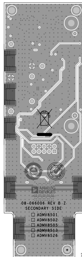
Figure 17. ADMV8502-EVALZ Layer 4
