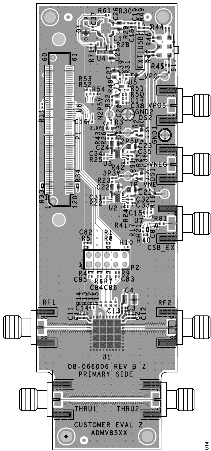
Figure 14. ADMV8502-EVALZ Layer 1
