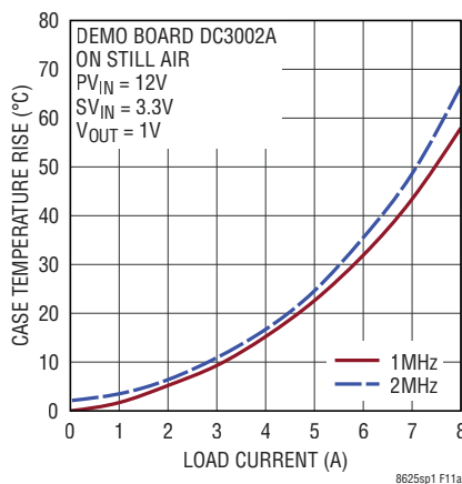
(a) LT8625SP
