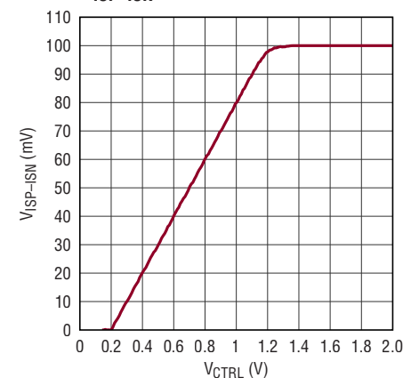
V_{SP-ISO} vs CTRL
