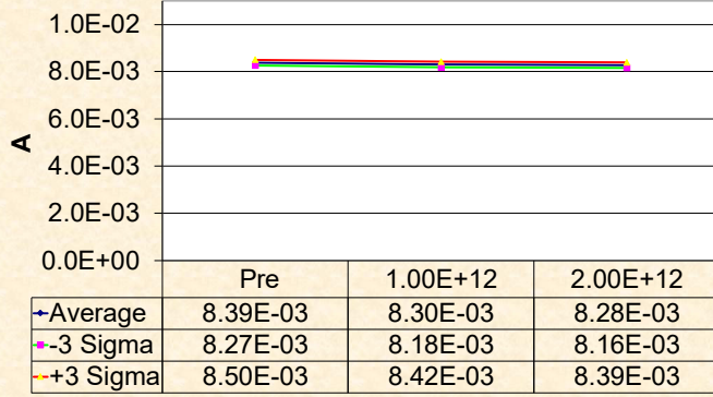
VIO Vcc=+/-15V Side A
