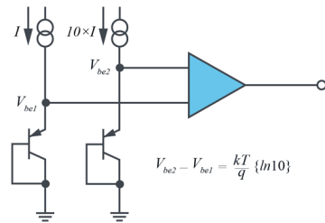
图1. 测量温度的基本电路。
