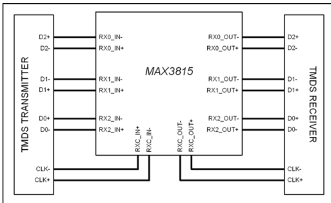
图 5. 连接方案
