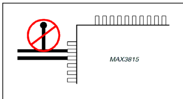
图 1. 存在不必要断线的 PCB 布局
