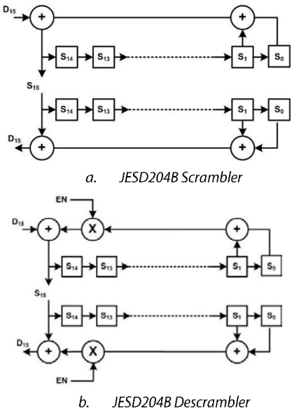
图4. JESD204B加扰/解扰
