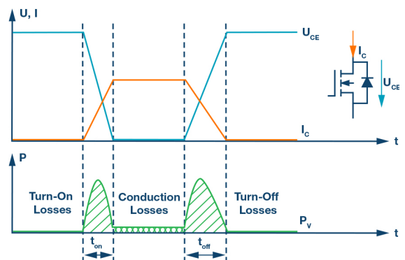
图2. 晶体管各个损耗分量的简化表示。
