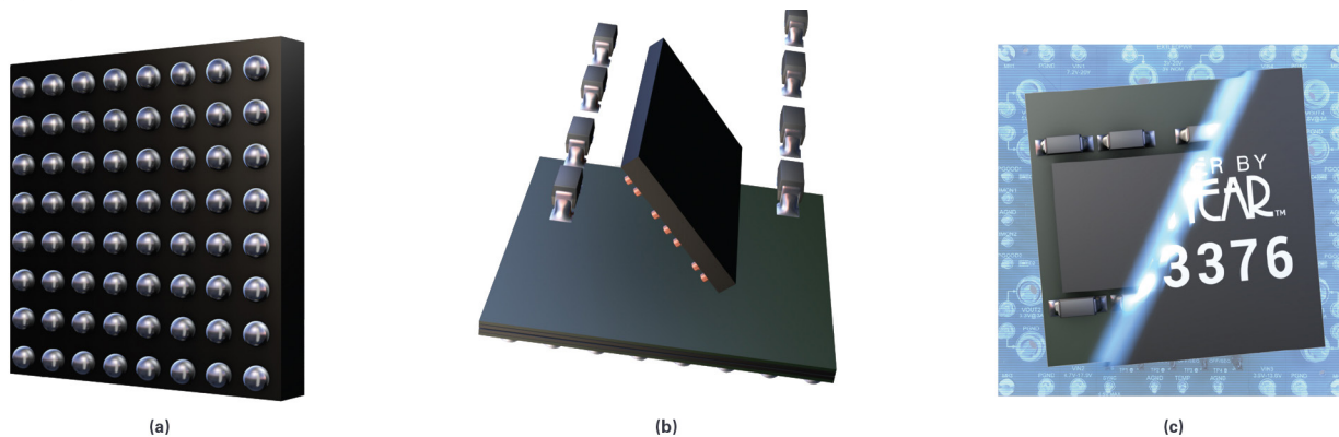
图3. LTC3376倒装封装(a)引脚球栅阵列, (b)铜柱在裸片下方以及(c)集成旁路电容。
