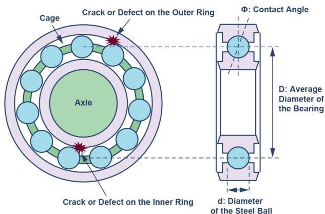
图4. 滚珠轴承。
