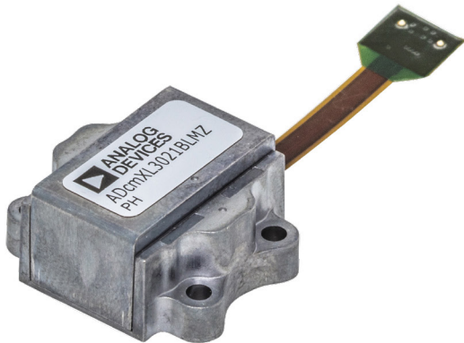
图2. ADcmXL3021模块，非常适合用于实施预测性维护。
