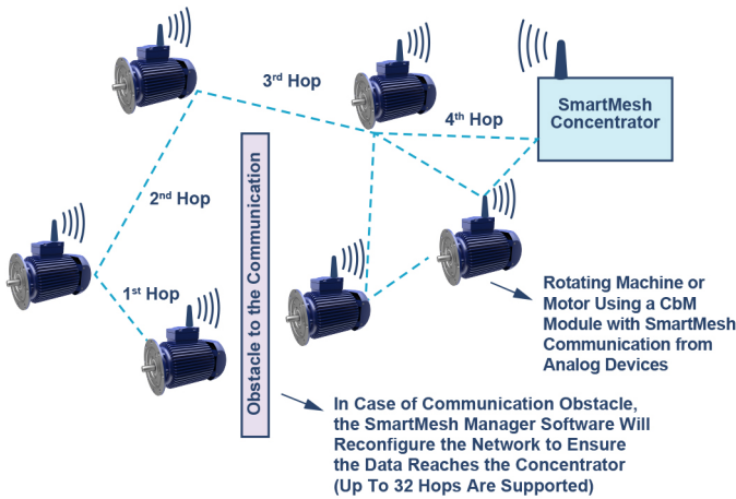
图3. SmartMesh IP网络非常适合用于实施IIoT和预测性维护操作。
