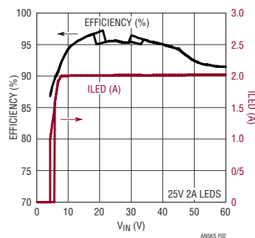
图 2：(a) 图 1 所示 50W LED 驱动器的效率在典型的 9V 至 16V 汽车电池输入范围内具有 98% 的峰值和 95% 至 97% 的变化范围。(b) LT8391 峰值电感器电流限制能够在低 V_{IN} 条件下通过降低输出功率以保持稳定性。
