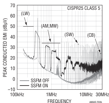
图 3：SSFM 把 LT8391 峰值和平均 EMI 降至低于 CISPR25 Class 5 限值。平均 EMI 的降幅比峰值 EMI 的降幅更大。
