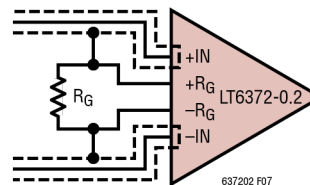
图6. 保护环可用于最大限度地减少进入输入引脚的漏电流
