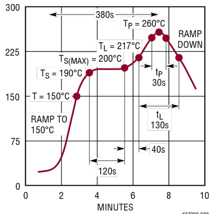
IR回流引起的无铅回流温度曲线
