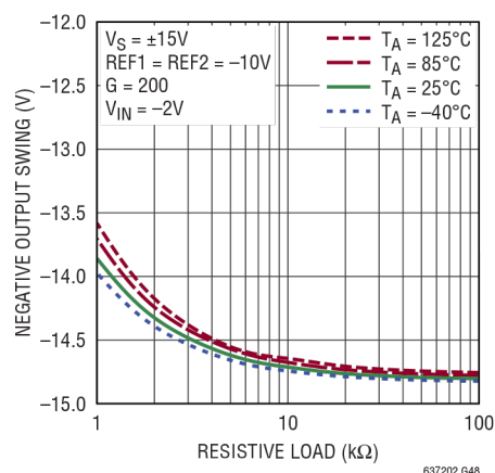
负输出摆幅与阻性负载的关系
