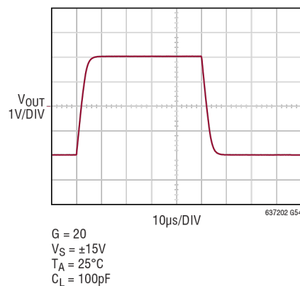
大信号瞬态响应
