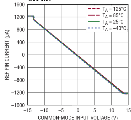
REF引脚电流与输入共模电压 的关系
