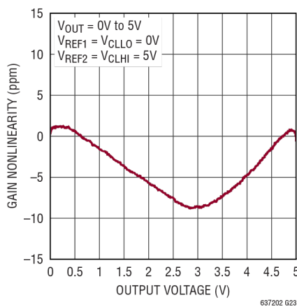
增益非线性( G = 10 )
