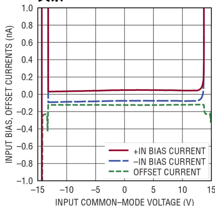
输入偏置电流与共模电压的 关系
