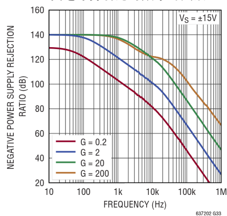
负电源抑制比与频率的关系
