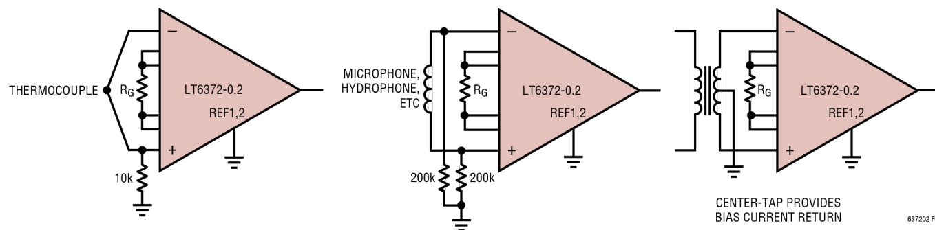
图7. 提供输入共模电流路径
