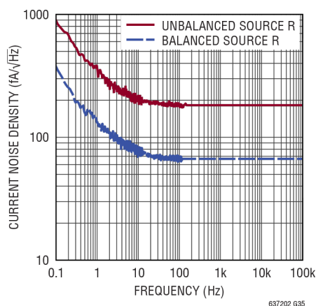
电流噪声密度与频率的关系
