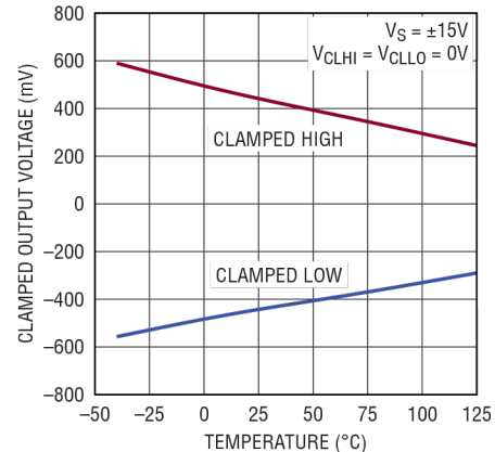
箝位电压与温度
