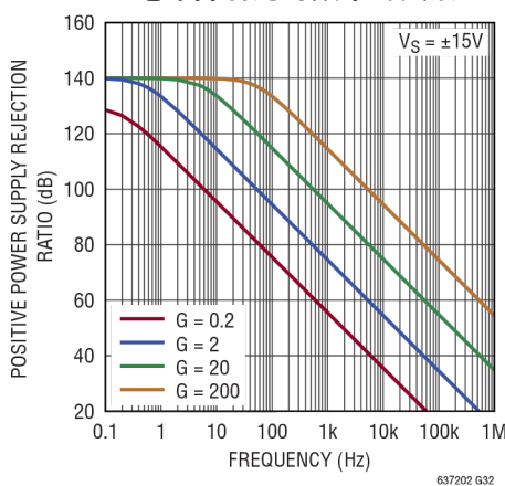
正电源抑制比与频率的关系
