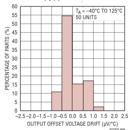
输出失调电压漂移分布图, MS16E封装
