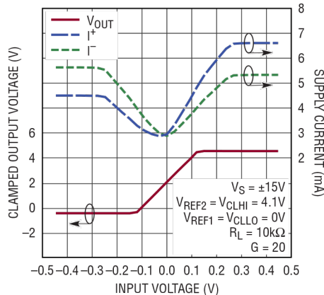
箝位时的电源电流
