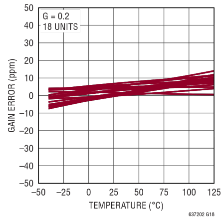
增益漂移(G = 0.2)
