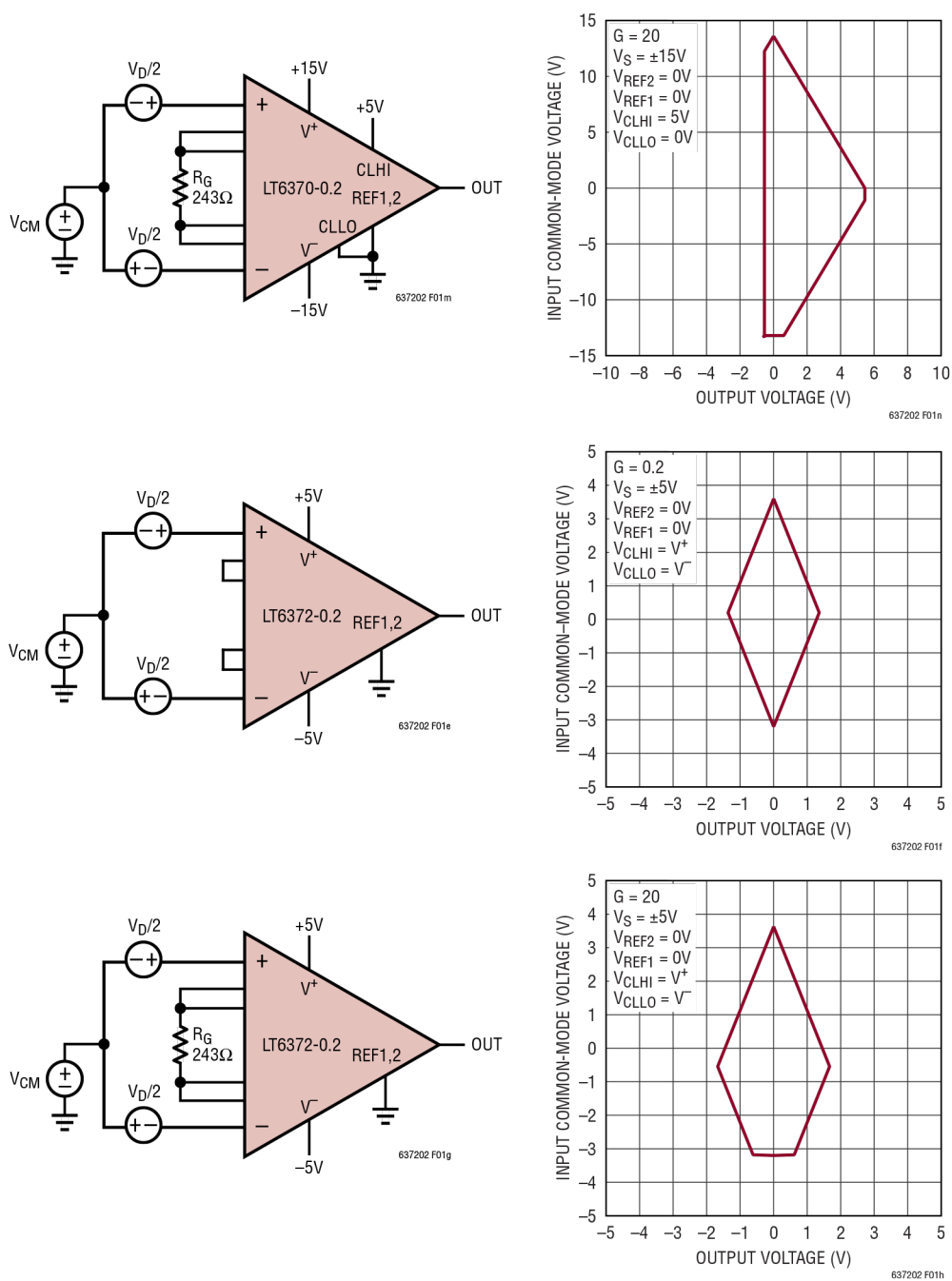
图1 (续) . 输入共模范围与输出电压的关系
