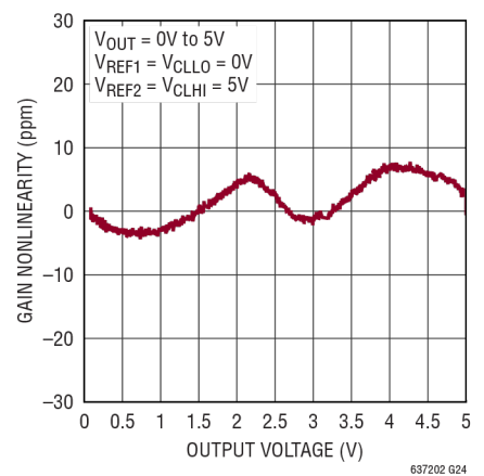
增益非线性( G = 100 )
