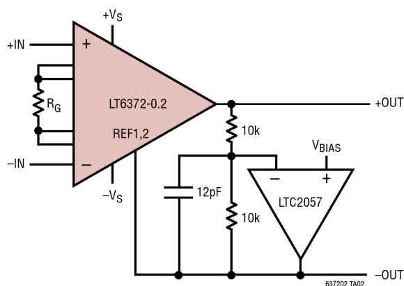
差分输出仪表放大器
