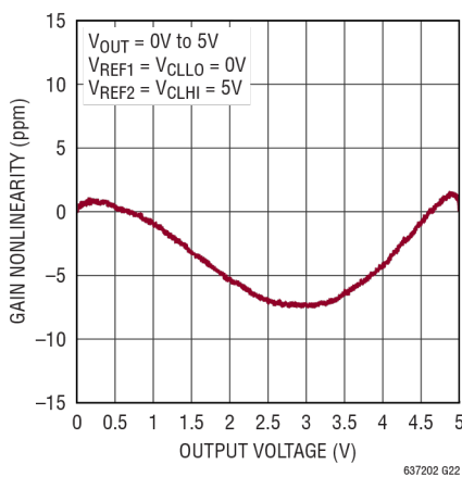
增益非线性( G = 1 )
