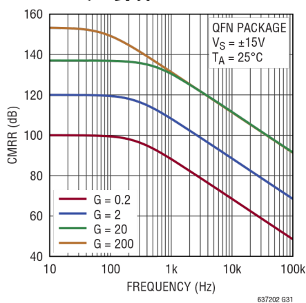
CMRR与频率的关系, RTI QFN封装
