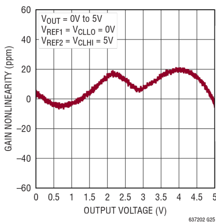
增益非线性( G = 200 )
