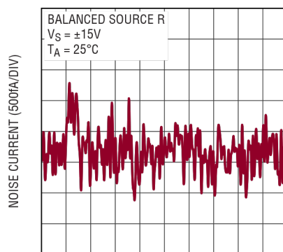
0.1Hz至10Hz噪声电流, 平衡源R
