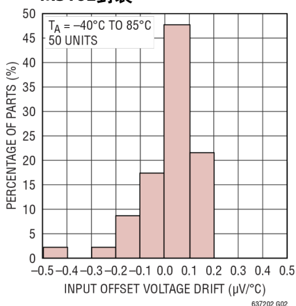
输入失调电压漂移分布图, MS16E封装
