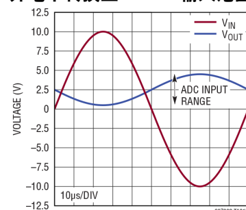
LT6372-0.2 衰减 \pm 10\text{V} 输入 并电平转换至 5\text{V} ADC 输入范围
