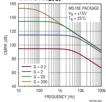
CMRR与频率的关系, RTI MS16E封装
