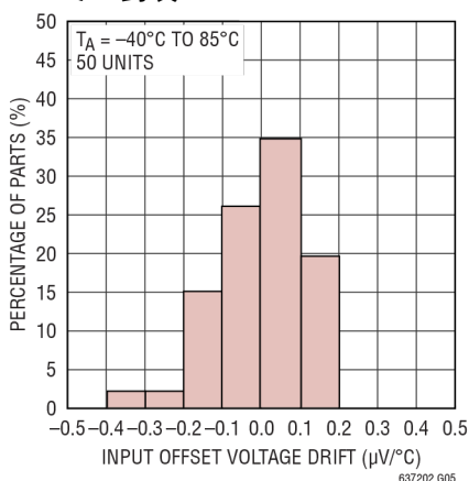
输入失调电压漂移分布图, QFN封装
