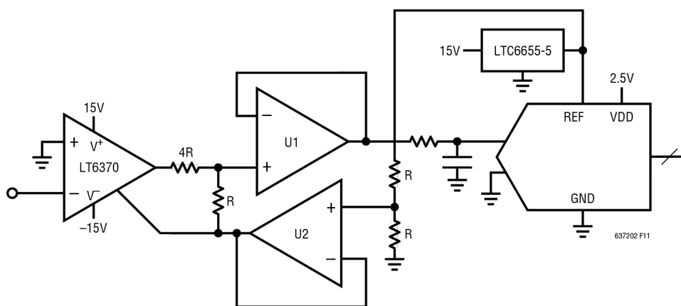
图11. 替代IA-ADC接口电路
