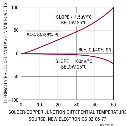
图4. 焊锡铜的热EMF
