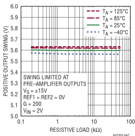
正输出摆幅与阻性负载的关系
