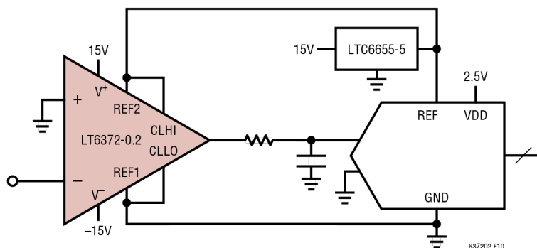
图10. LT6372-0.2集成ADC驱动解决方案
