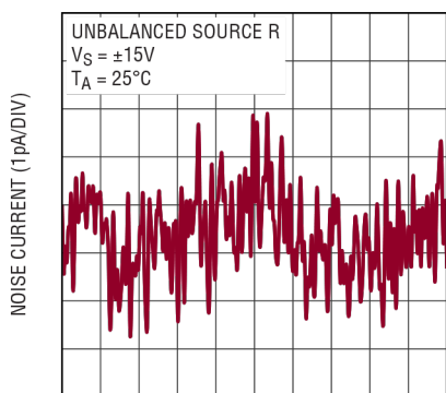
0.1Hz至10Hz噪声电流, 非平衡源R
