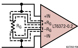
图5. 保护环可用于最大限度地减少进入 R_G 引脚的漏电流
