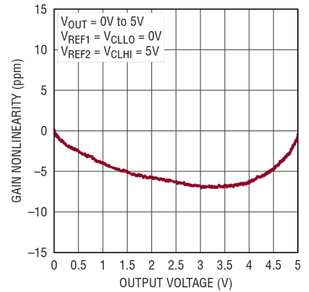
增益非线性( G = 0.2 )
