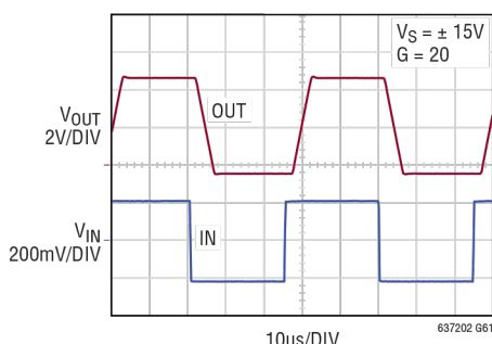
箝位瞬态响应
