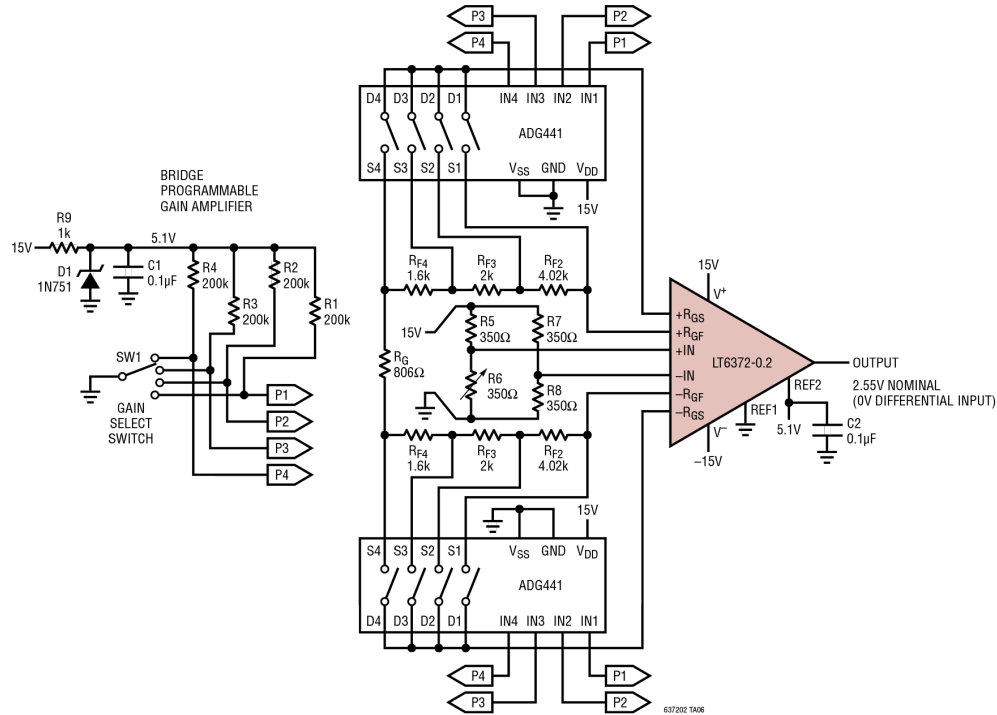
增益为0.5V/V、1V/V、2V/V和10V/V的可编程增益放大器
