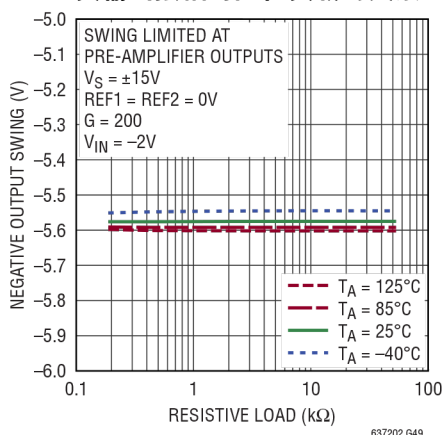
负输出摆幅与阻性负载的关系
