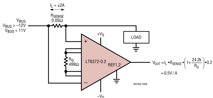
高端、双向电流检测
