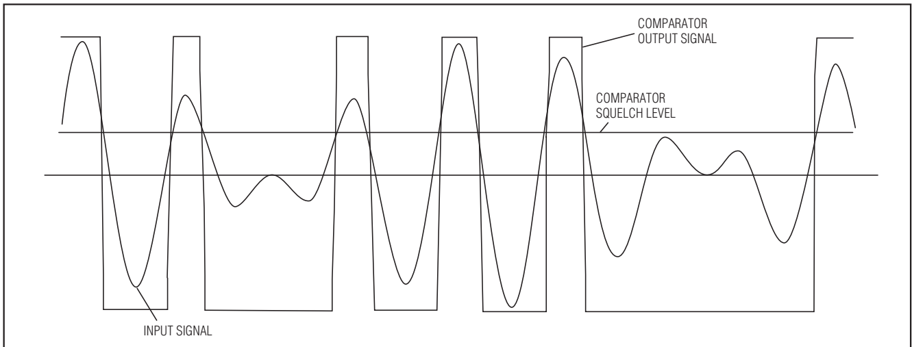
图6. 采用比较器时 \overline{\text{VIBE}} 的输出
