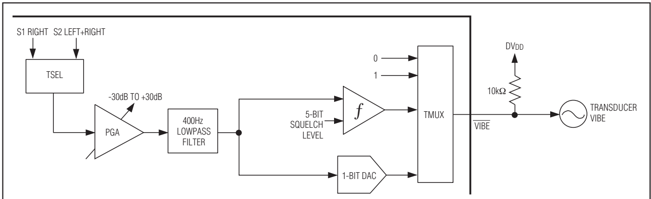
图7. 蜂鸣器/振动器功能框图
