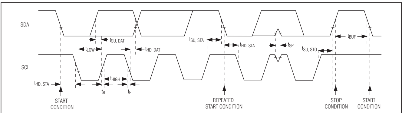
图10. 2线接口时序图
