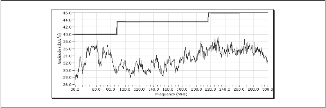
图2. SSM辐射
