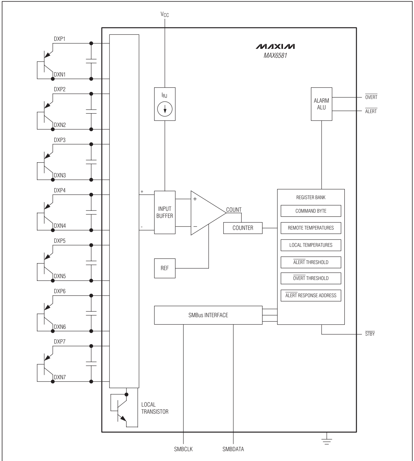
图1. 内部框图
