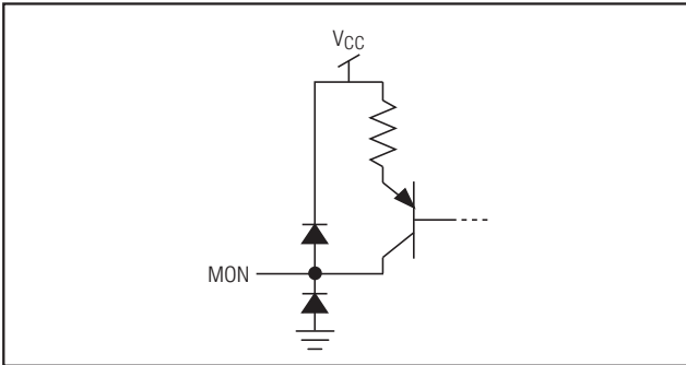
图8. MON接口
