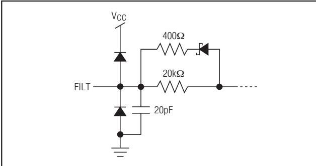
图7. FILT接口
