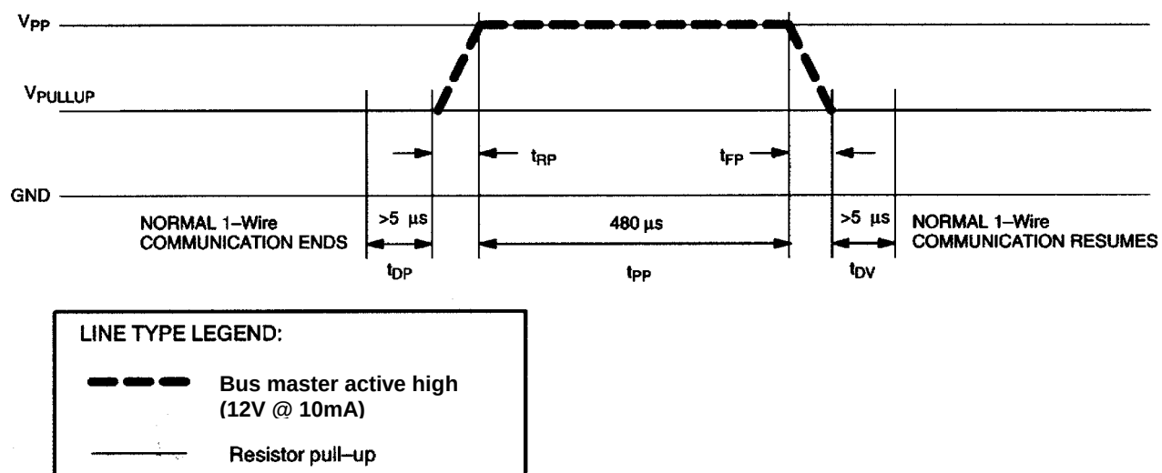
编程脉冲时序图 图 12
