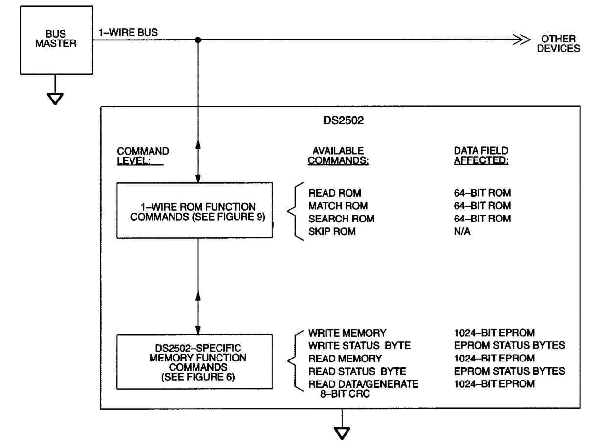
1-Wire 协议的层次结构图 图 2
