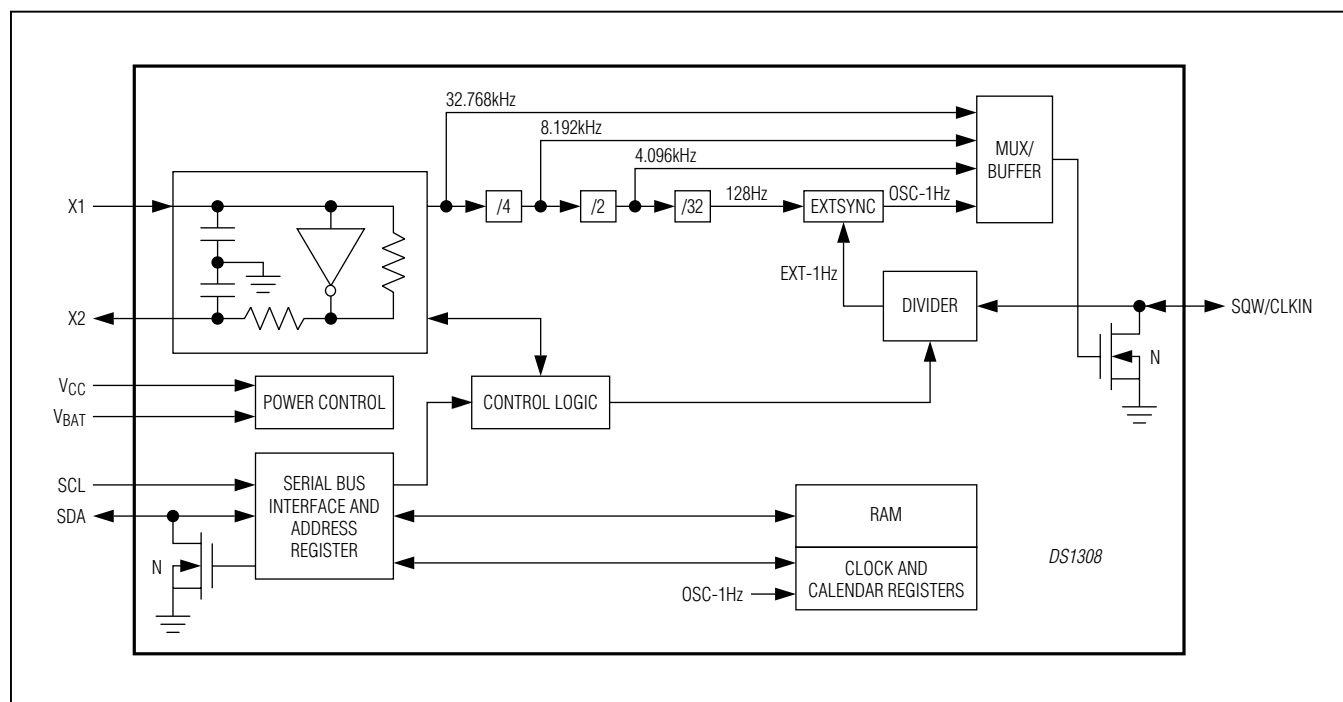
功能框图
